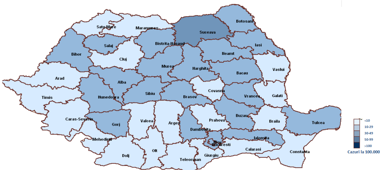
Incidenta aparenta (ultimele 14 zile) la 100.000 locuitori
